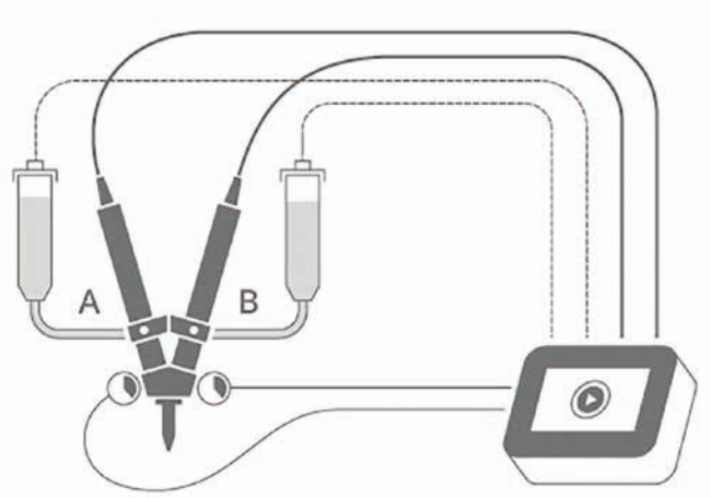
Liquides non autonivelants, fluide de moyenne à haute viscosité, y compris technologie des capteurs et pression d'entrée
