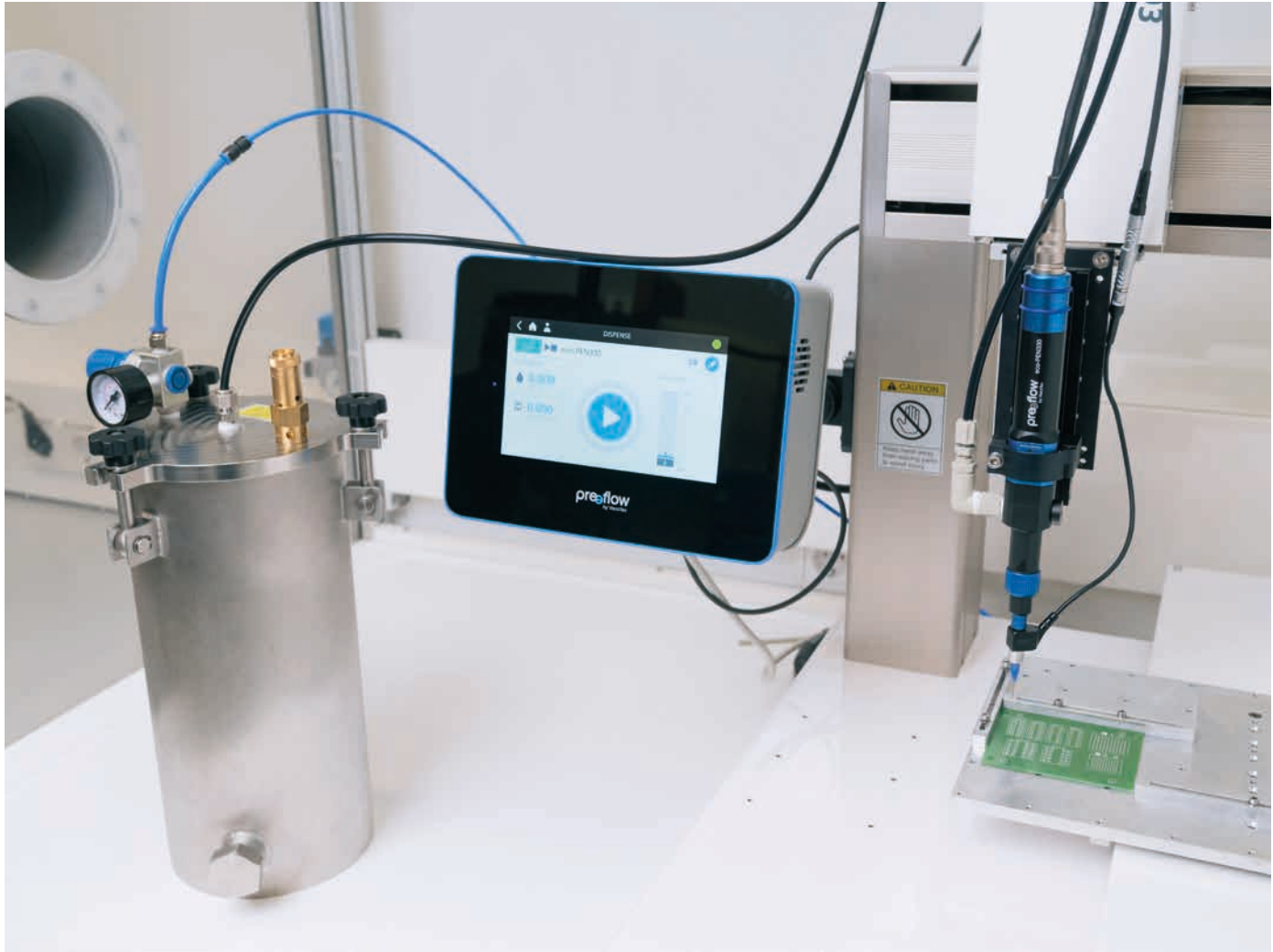
Constitution réelle du système
